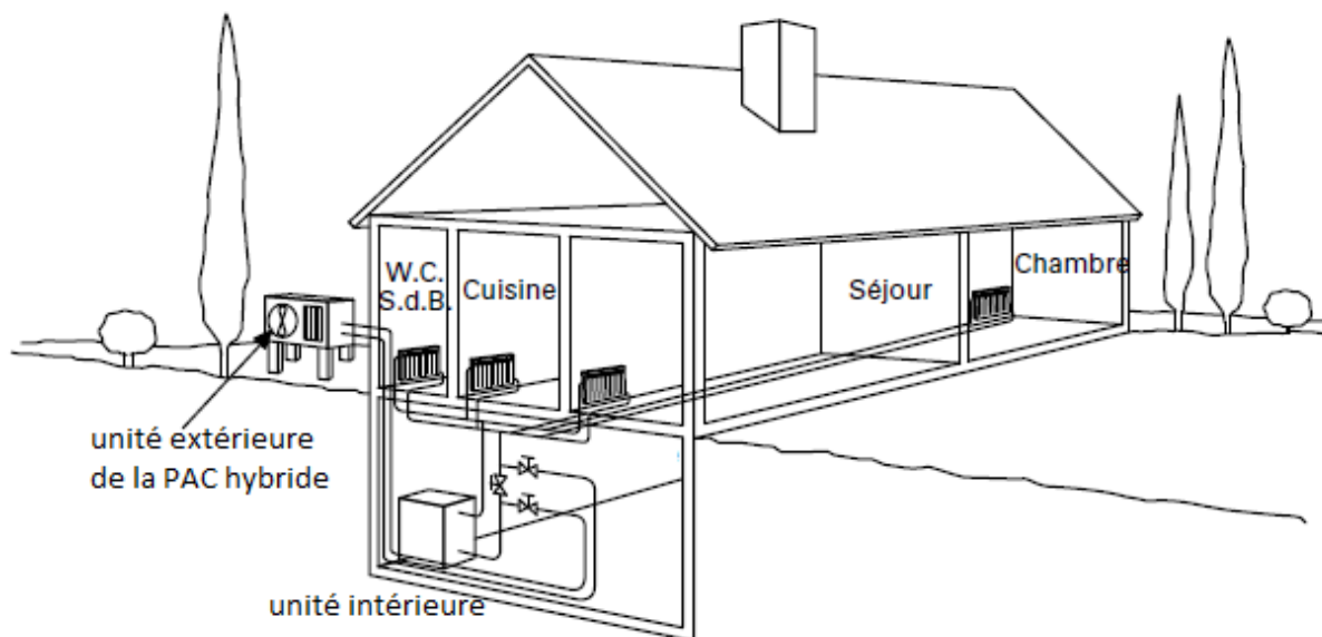
Figure 11 : Exemple de pompe à chaleur hybride
