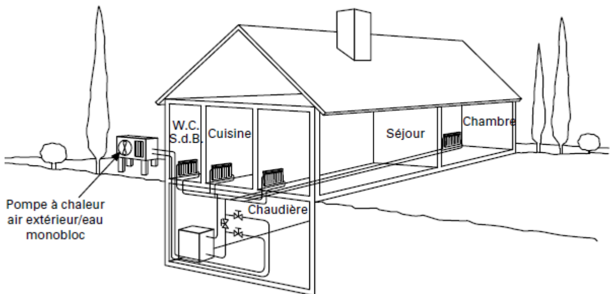
Figure 5 : Exemple de chaudière existante en relève de pompe à chaleur air extérieur-eau
