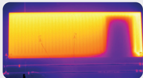
Thermographie infrarouge. Flèche -> zone froide.
