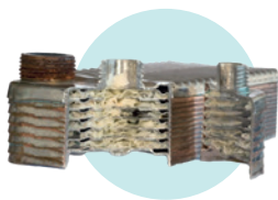
Échangeur entartré
